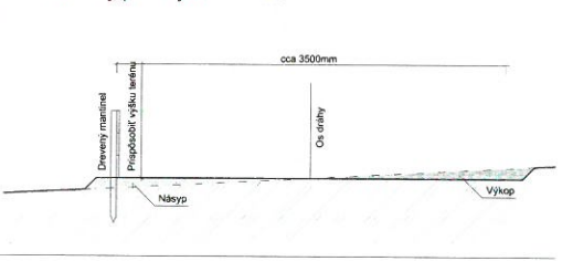
Schematicky priečný rez M 1:20
