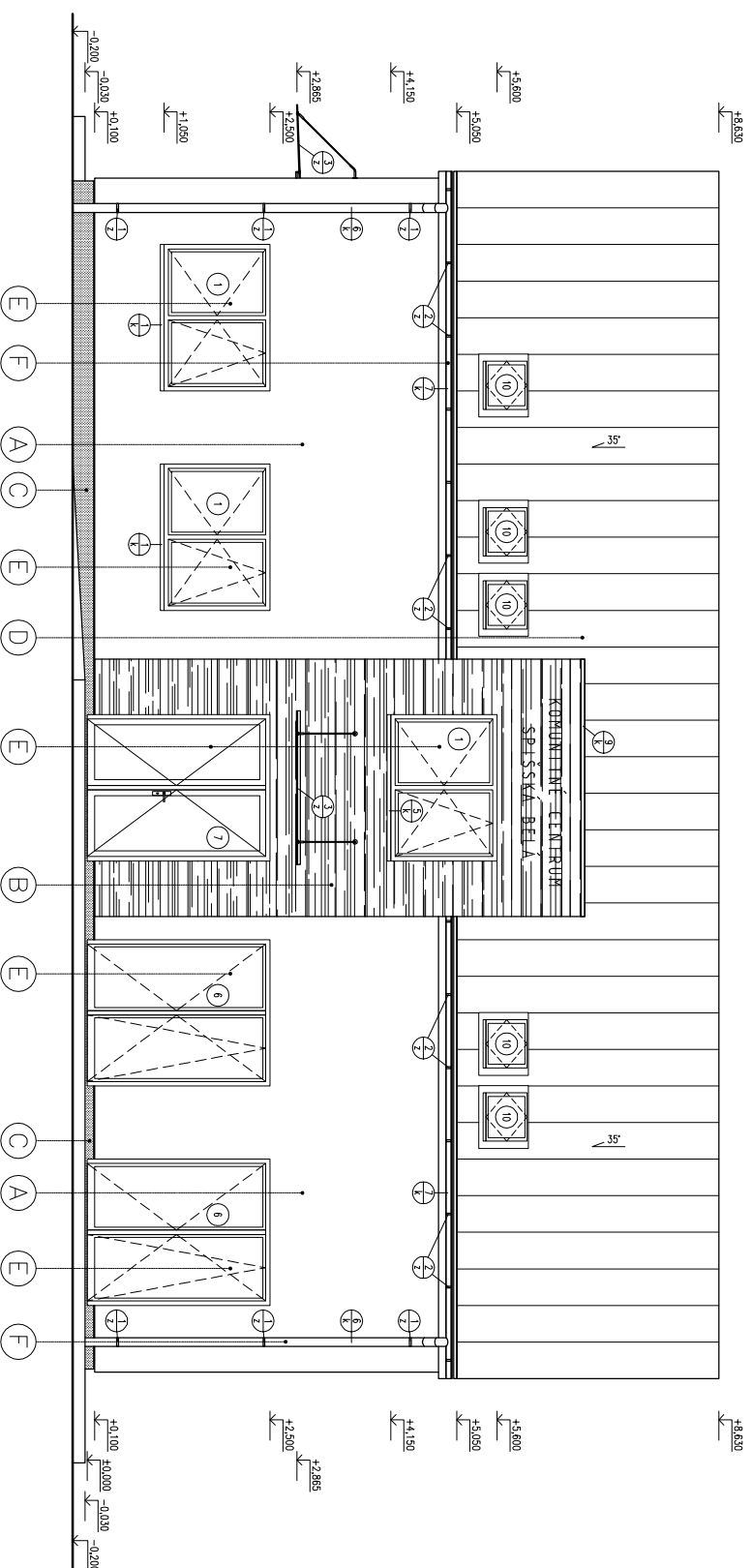
POHĽAD SEVEROZÁPADNÝ
