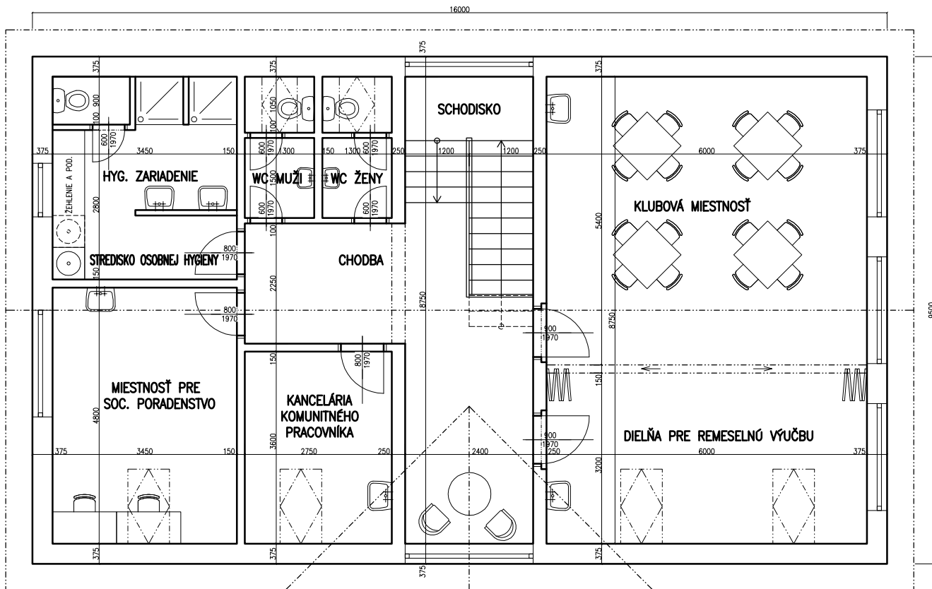
PÔDORYS 2.NP
