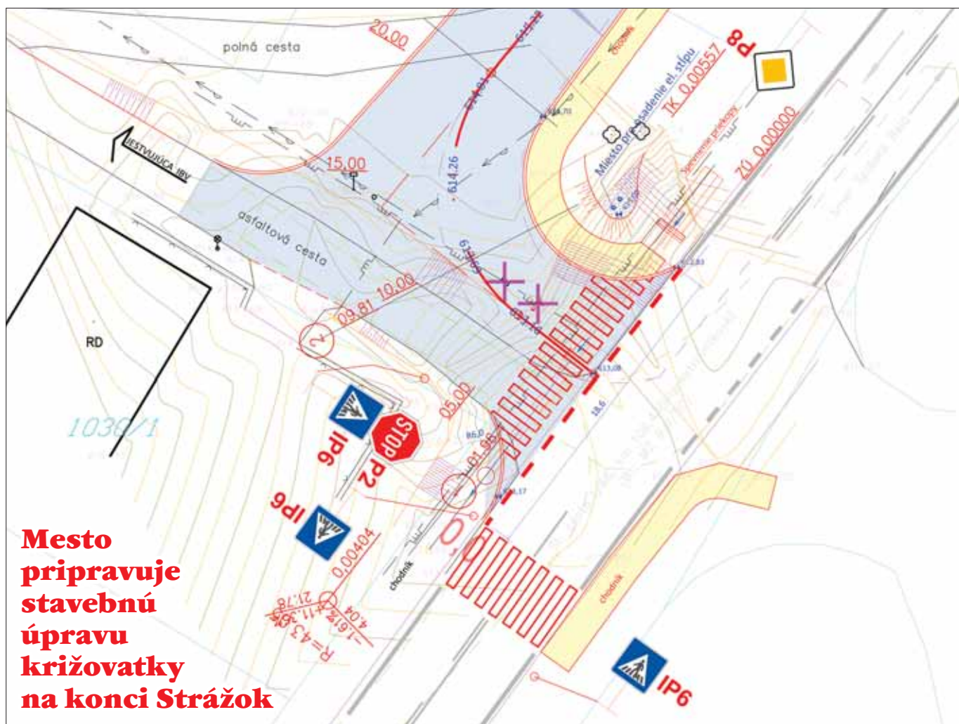
Parkovanie a zmena dopravy na Štefánikovej ulici - návrh riešenia
